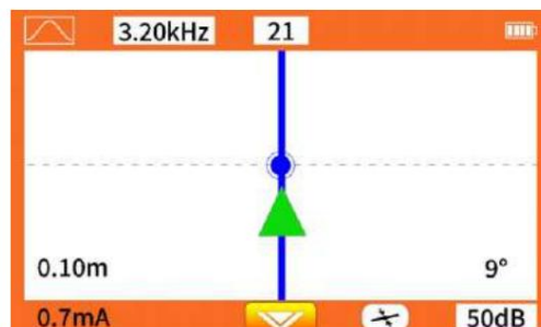
Modalità segnale a schermo intero
